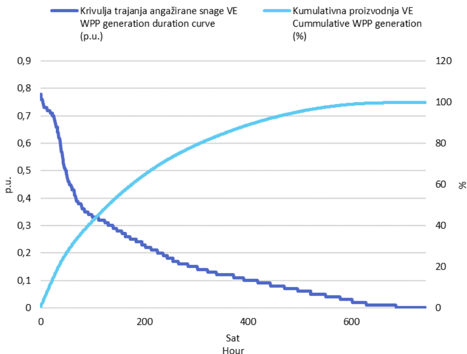
Slika 3 Krivulja trajanja angažirane snage svih VE i kumulativna proizvodnja VE u svibnju 2022. godine u jediničnim vrijednostima
