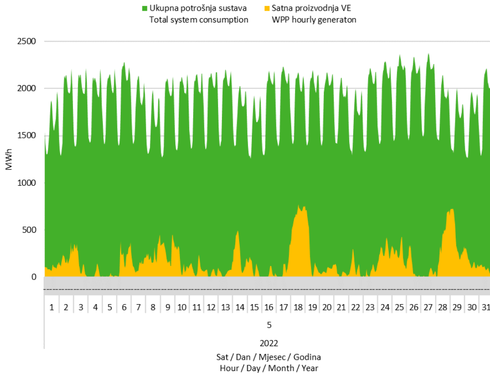
Slika 7 Usporedba satnog dijagrama opterećenja sustava i proizvodnje vjetroelektrana u svibnju 2022. godine
