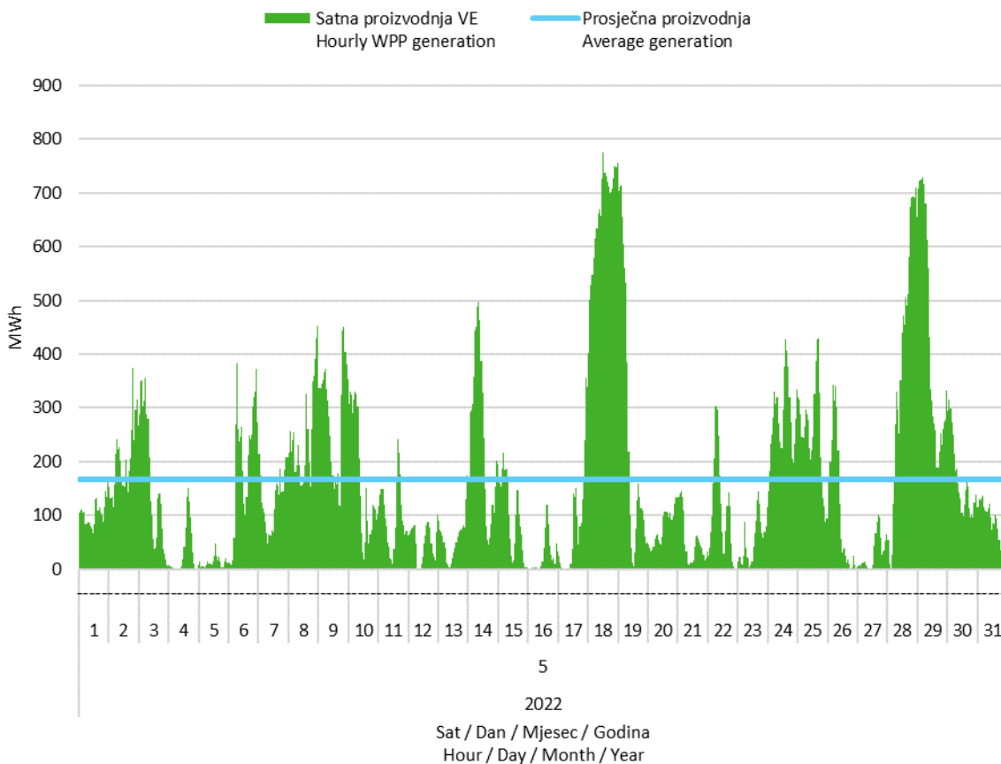
Slika 2 Satna proizvodnja svih vjetroelektrana u svibnju 2022. godine
