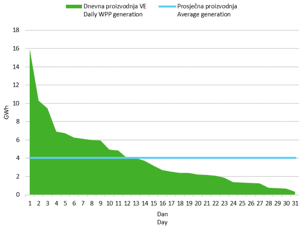
Slika 6 Krivulja trajanja dnevne proizvodnje vjetroelektrana u svibnju 2022. godine
