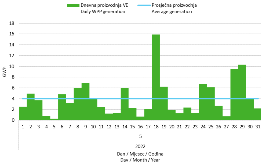
Slika 5 Dnevna proizvodnja svih vjetroelektrana u svibnju 2022. godine Figure 5 Daily generation of all wind power plants in May 2022
