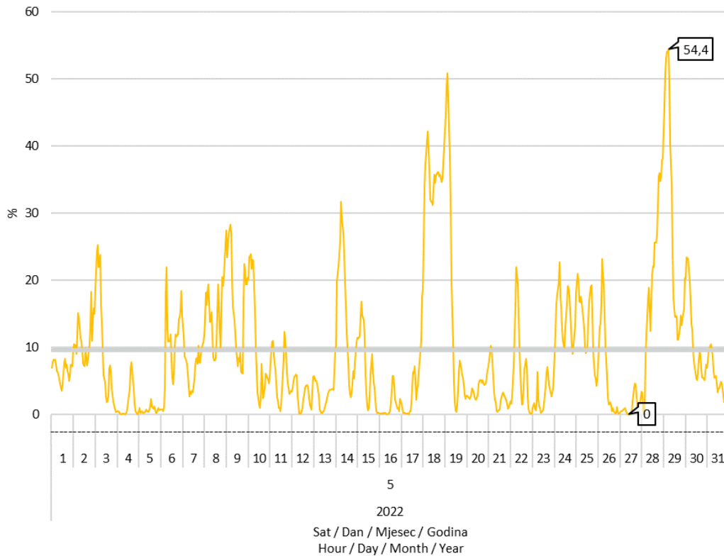
Slika 8 Udio proizvodnje vjetroelektrana u pokrivanju satnog opterećenja elektroenergetskog sustava u svibnju 2022. godine
