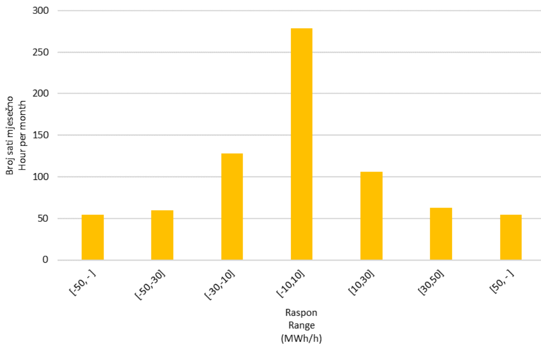
Slika 10 Statistička raspodjela satnih promjena proizvodnje VE u svibnju 2022. godine
