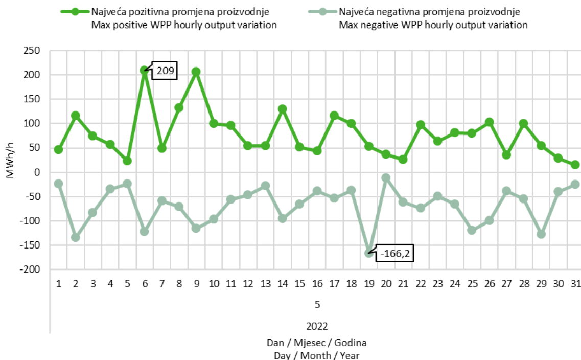
Slika 9 Maksimalna pozitivna i maksimalna negativna promjena satne proizvodnje VE u svibnju 2022. godine
